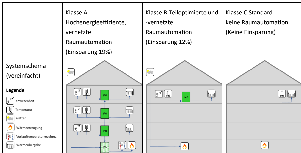
Abbildung 28: Vereinfachte Darstellung von System- und Automationsklassen für das Energiemanagement in Gebäuden
